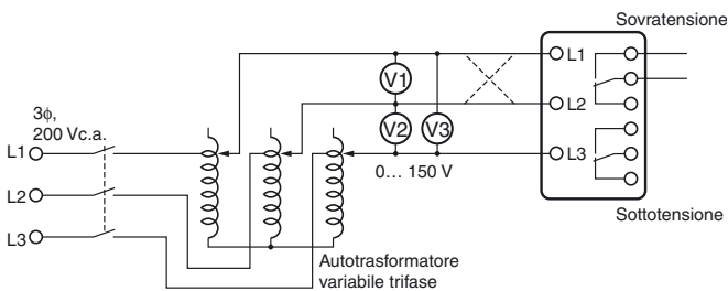
Schema di collegamento 1
